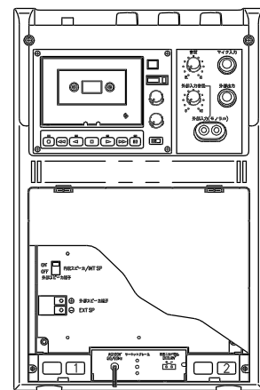
背面図
