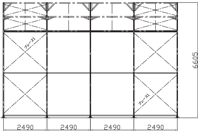
A-B 通り図
