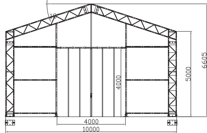
①-⑤ 通り図
