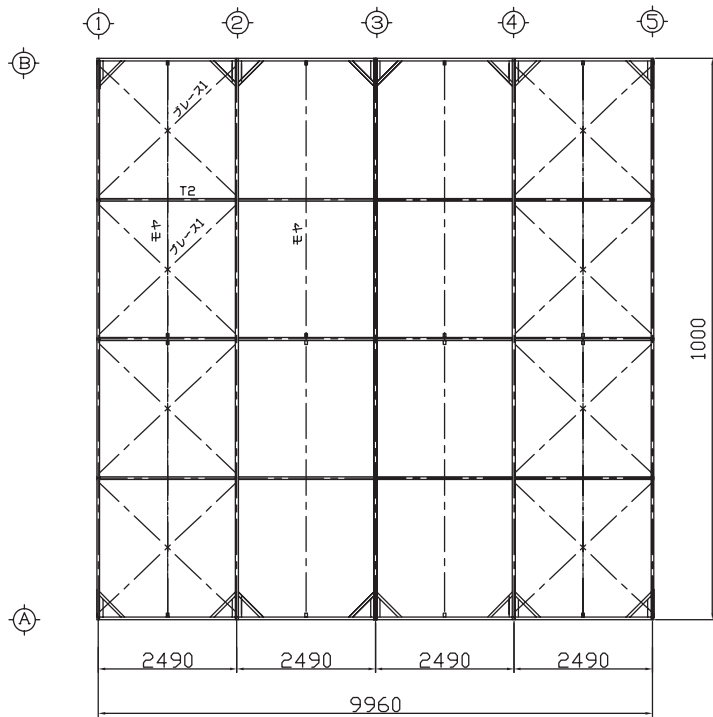
梁伏せ図
