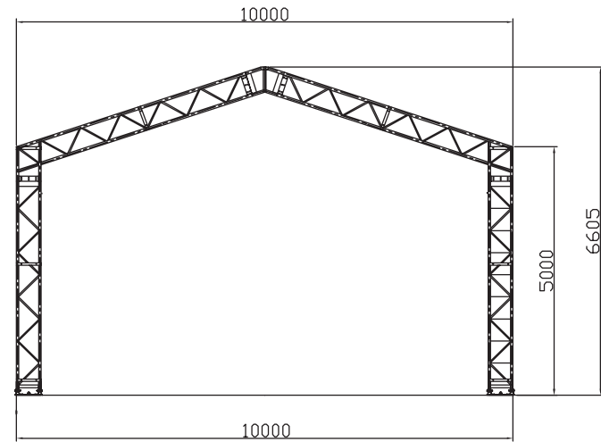
②-③-④ 通り図
